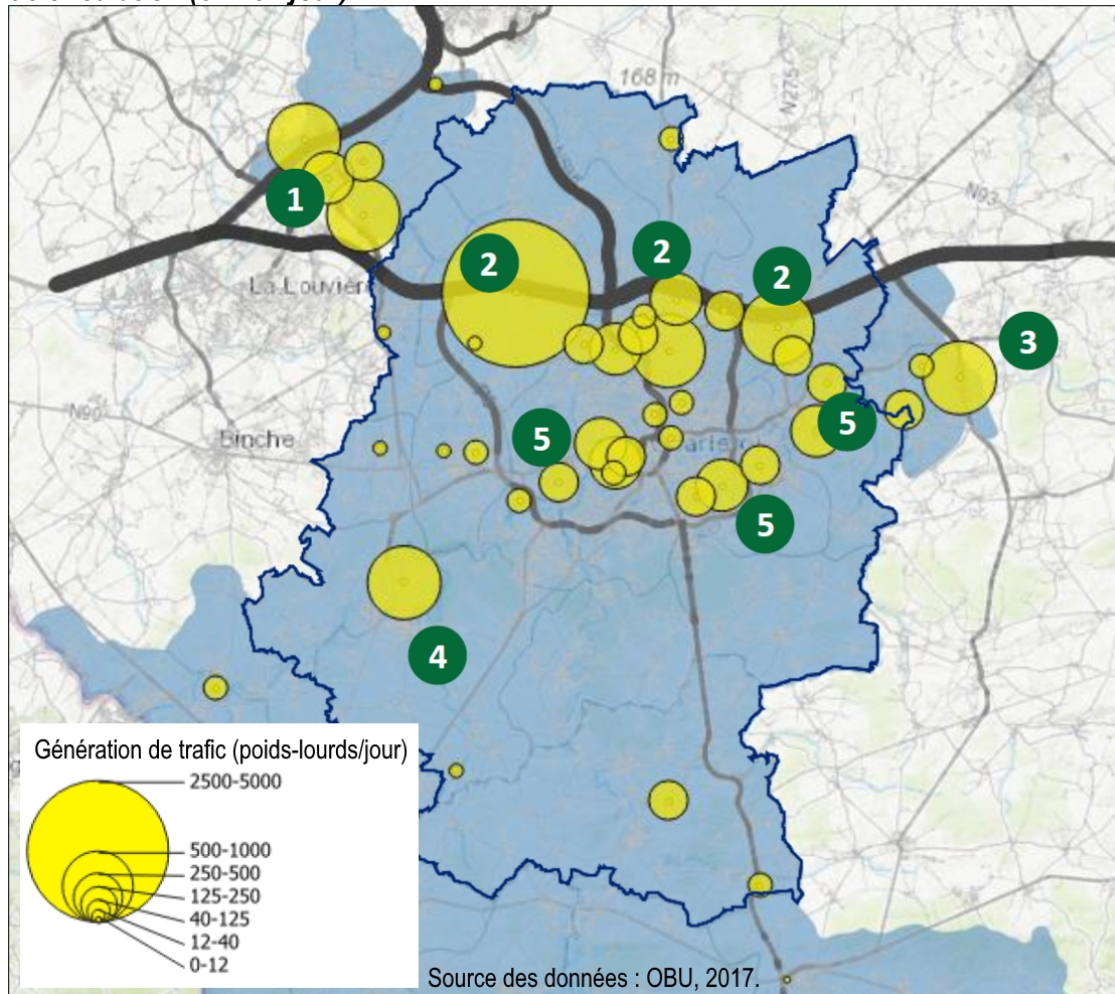
Illustration IV.7.18. Flux de véhicules de plus de 3,5 t pour un jour ouvrable et par sens de circulation (en véh/jour).
