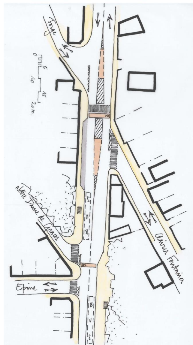
Esquisse : Carrefour N584 / rue de l'Épine
